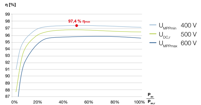
PIKO MP plus 3.0 bis 5.0 mit 2 MPP Tracker
